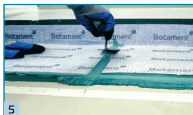
5 Izolační pás PB na spoji přesadit nejméně o 5 cm.
