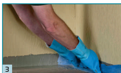
3 Zapracování izolačního pásu SB78, a hotových prvků v koutech a nárožích, do stěrky MD1 Speed nebo Multiproof.
